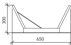
■ Legnaia MEZZO ESAGONO Art. GA LE.020
