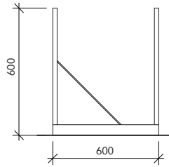
■ Legnaia RETTANGOLO Art. GA LE.015
