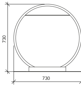
■ Legnaia CERCHIO Art. GA LE.027
