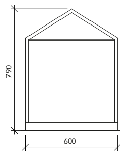
■ Legnaia CASA Art. GA LE.029
