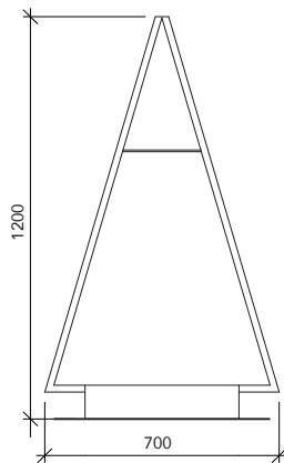
■ Legnaia MEZZO ESAGONO Art. GA LE.020
