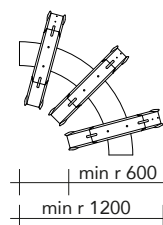
Mod. H 27 Support circulaire 1/4
