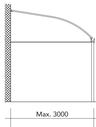
Vue latérale
