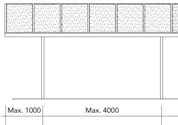
Vue frontale
