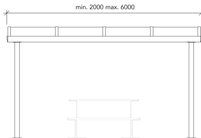
VISTA LATERALE
