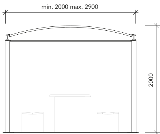
VISTA FRONTALE
